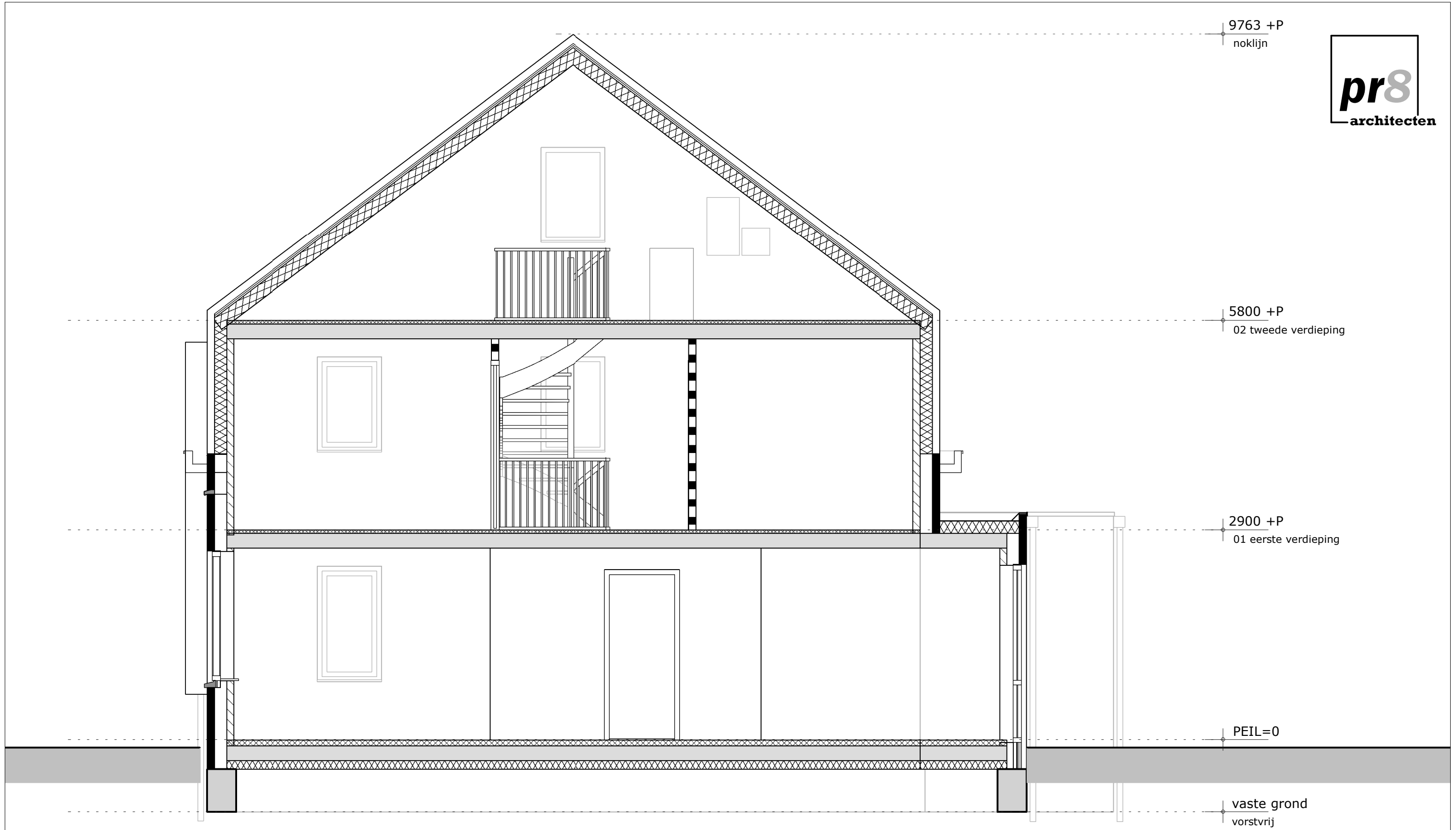
doorsnede B-B
